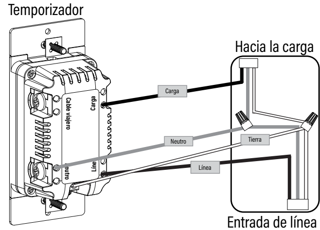
Cableado monopolar típico
