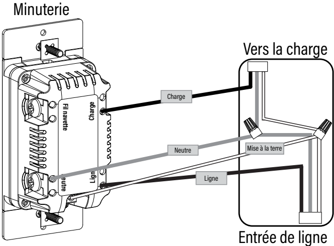
Câblage unipolaire typique
